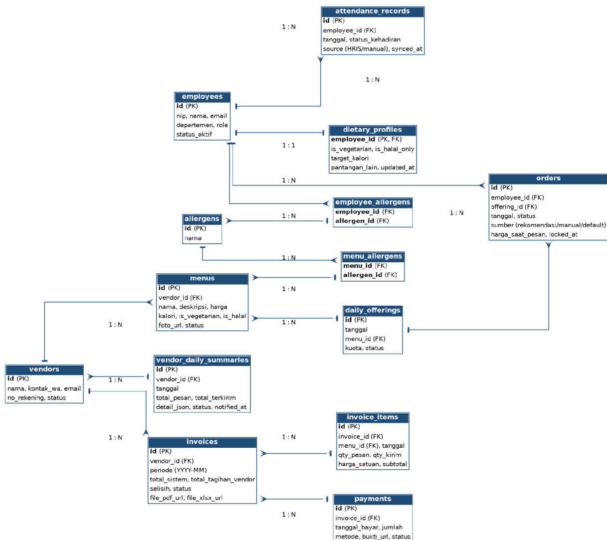
Gambar 7.1. ERD dengan 14 tabel domain utama.
