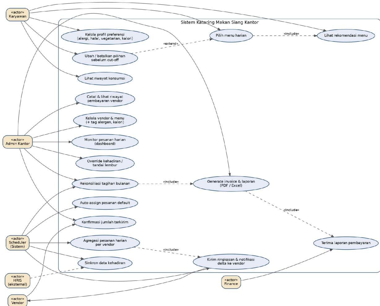
Gambar 9.1. Use case diagram dengan enam aktor.
